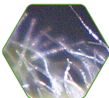
MÉLANGE CLASSIQUE
